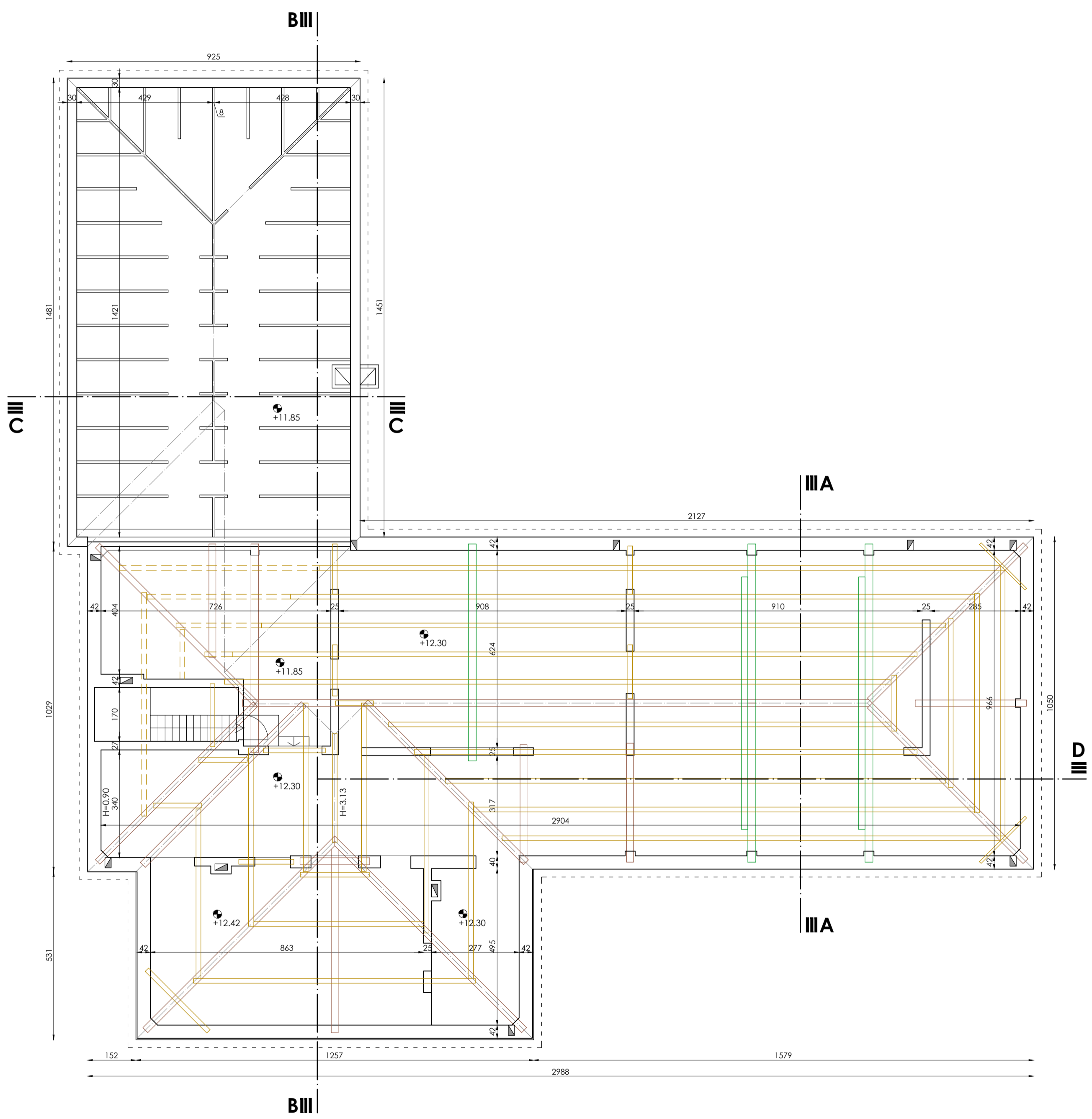
PIANTA ORDITURA COPERTURA
