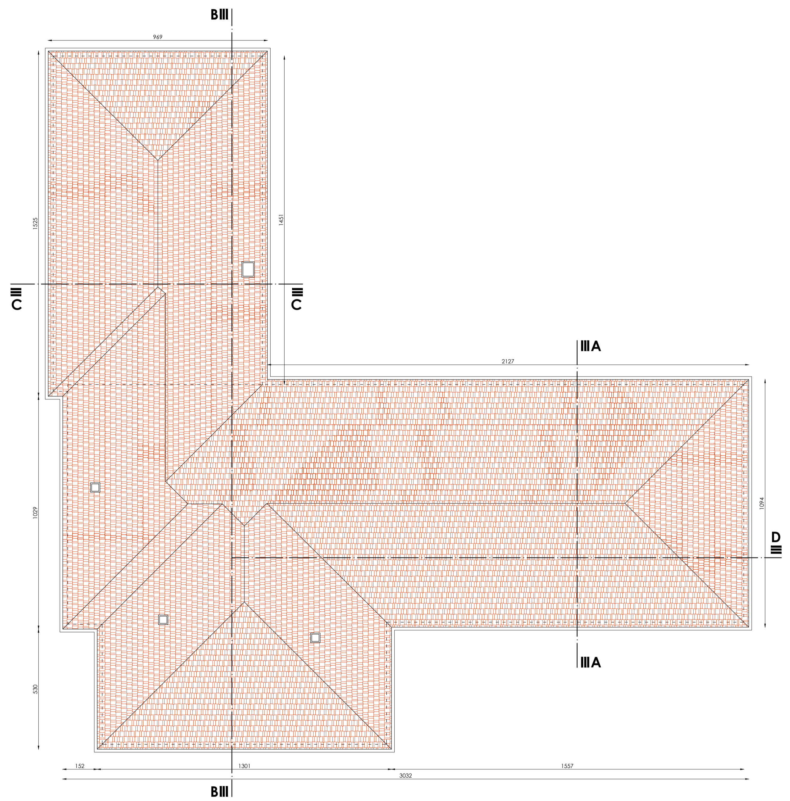
PIANTA COPERTURA
