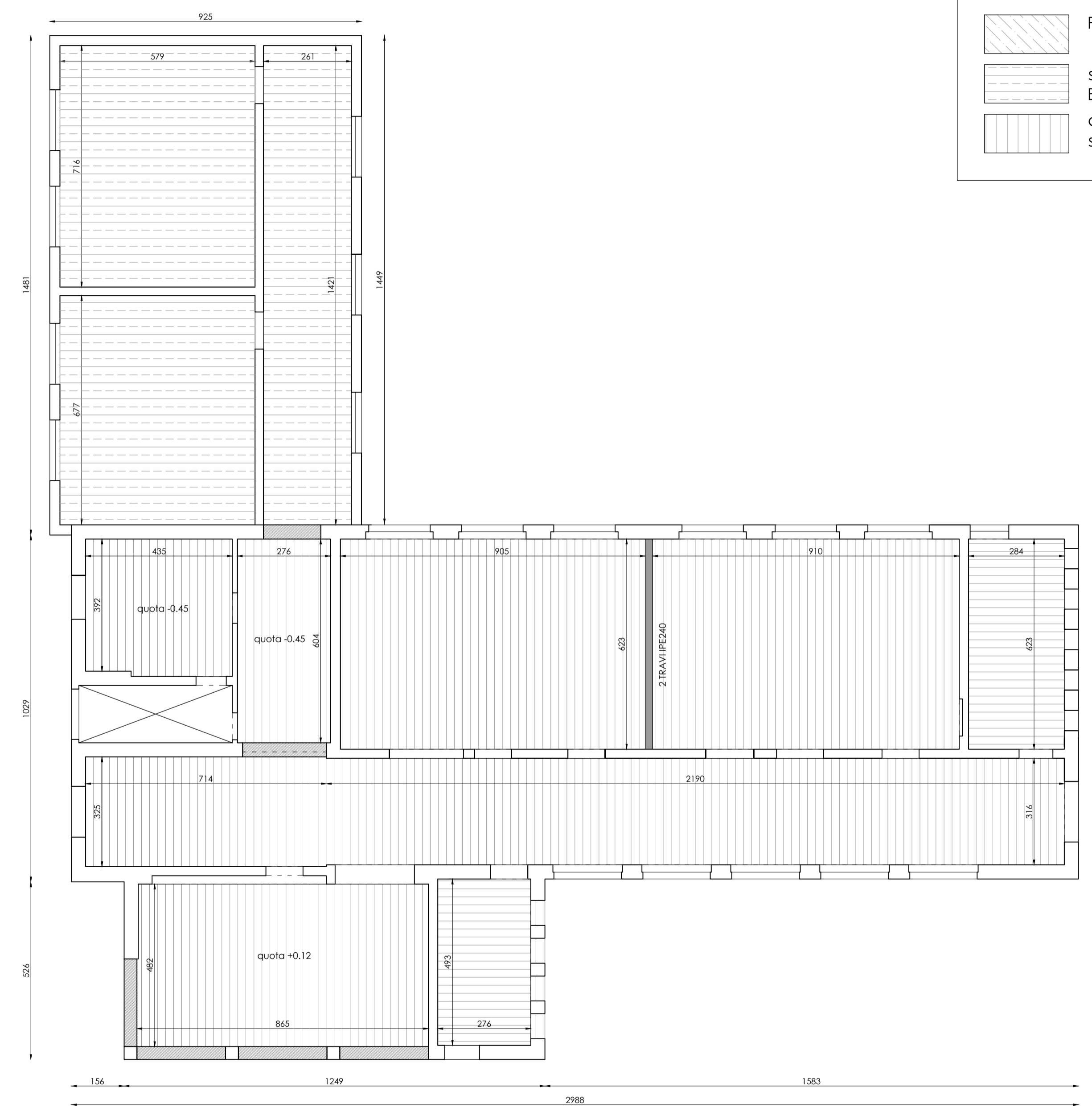
PIANTA TERZO SOLAIO
