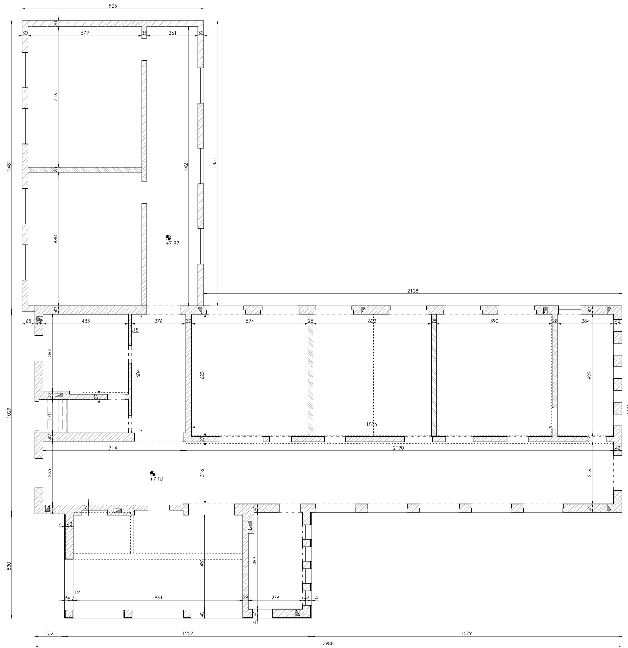
PIANTA MURATURE PIANO PRIMO
